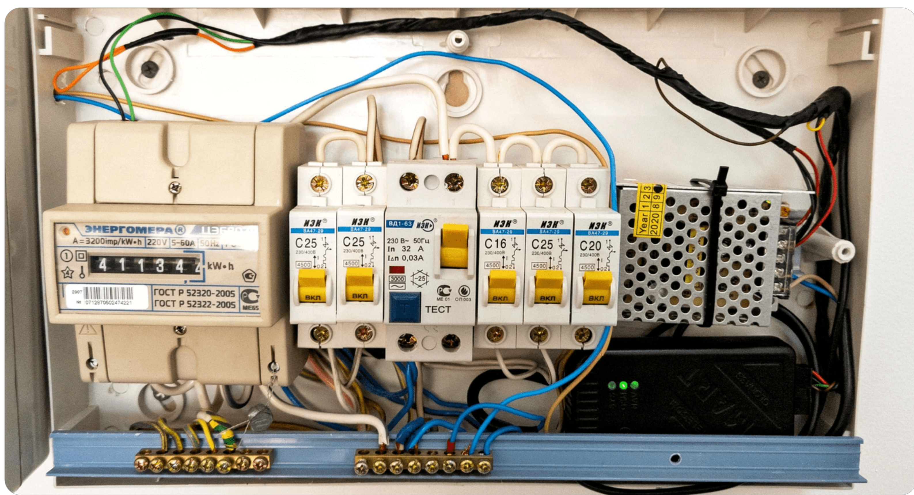
МОНИТОРИНГОВЫЙ ТЕРМИНАЛ, УСТАНОВЛЕННЫЙ В ЩИТЕ С ЭЛЕКТРОСЧЕТЧИКАМИ
